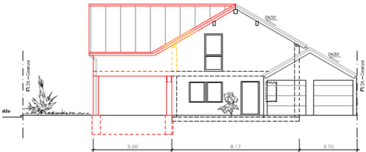
Ansicht Süd – aktualisierte Planung
