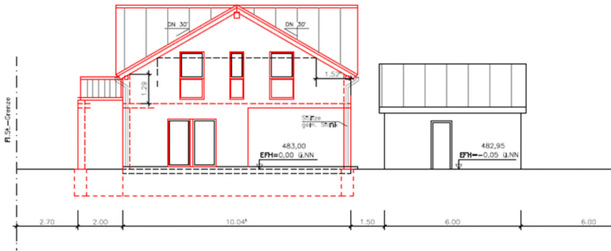
Ansicht West – aktualisierte Planung
