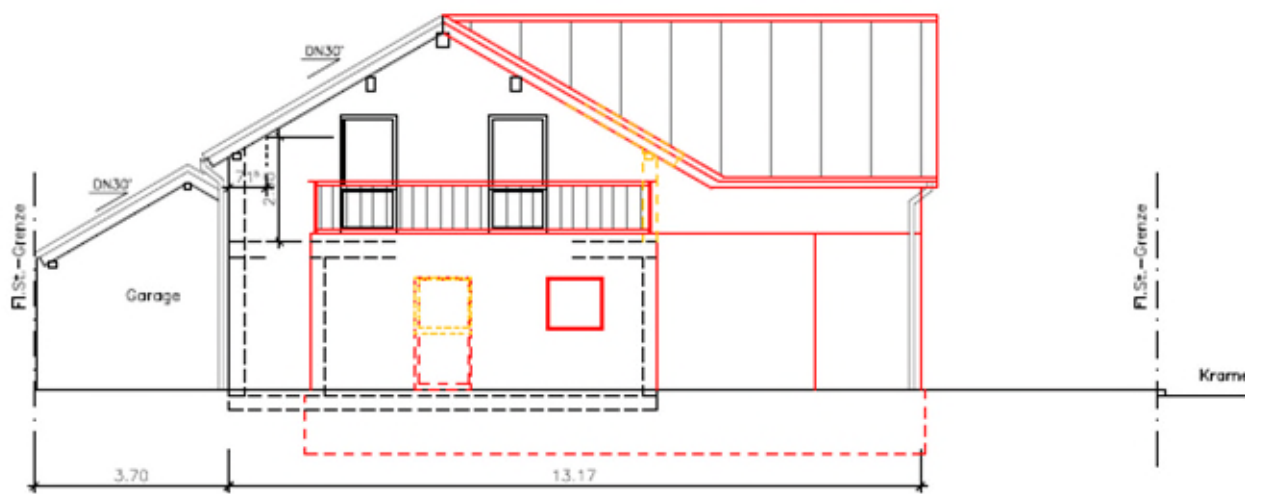
Ansicht Nord – aktualisierte Planung
