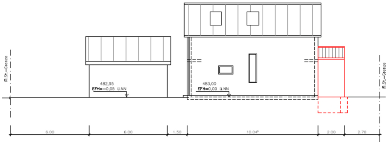
Ansicht Ost – ursprüngliche Planung
