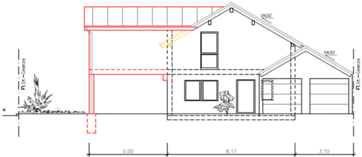
Ansicht Süd – ursprüngliche Planung
