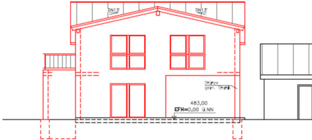
Ansicht West – ursprüngliche Planung
