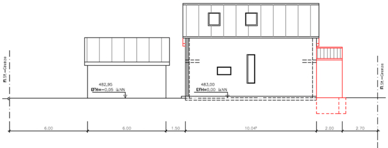
Ansicht Ost – aktualisierte Planung
